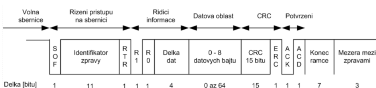
Obr. 12.4 Datová zpráva podle specifikace CAN 2.0A [12.2]
