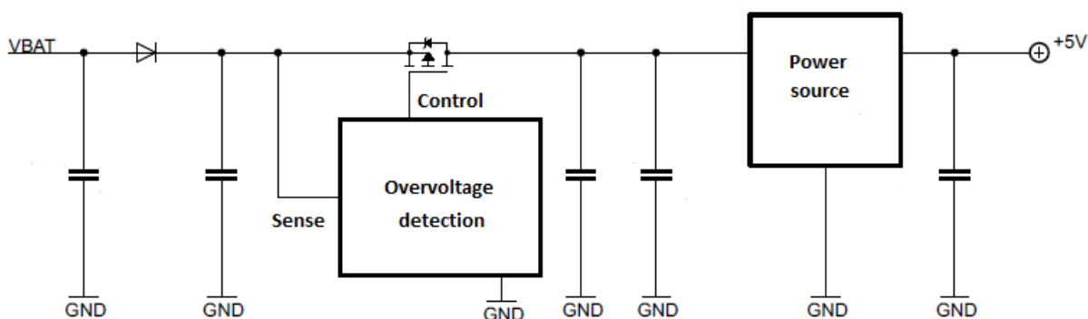
Obr. 11.5 Ochrana odpojením
