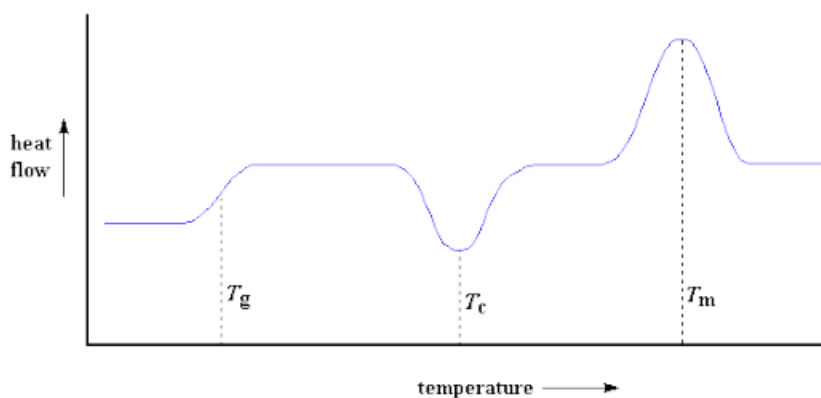
Obr. 5.6 Schematické znázornění DSC analýzy: T_g – teplota skelného přechodu, T_c – teplota krystalizace a T_m – teplota tavení [5.17]
