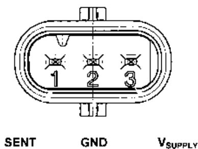
Obr. 12.6 Konektor snímače
