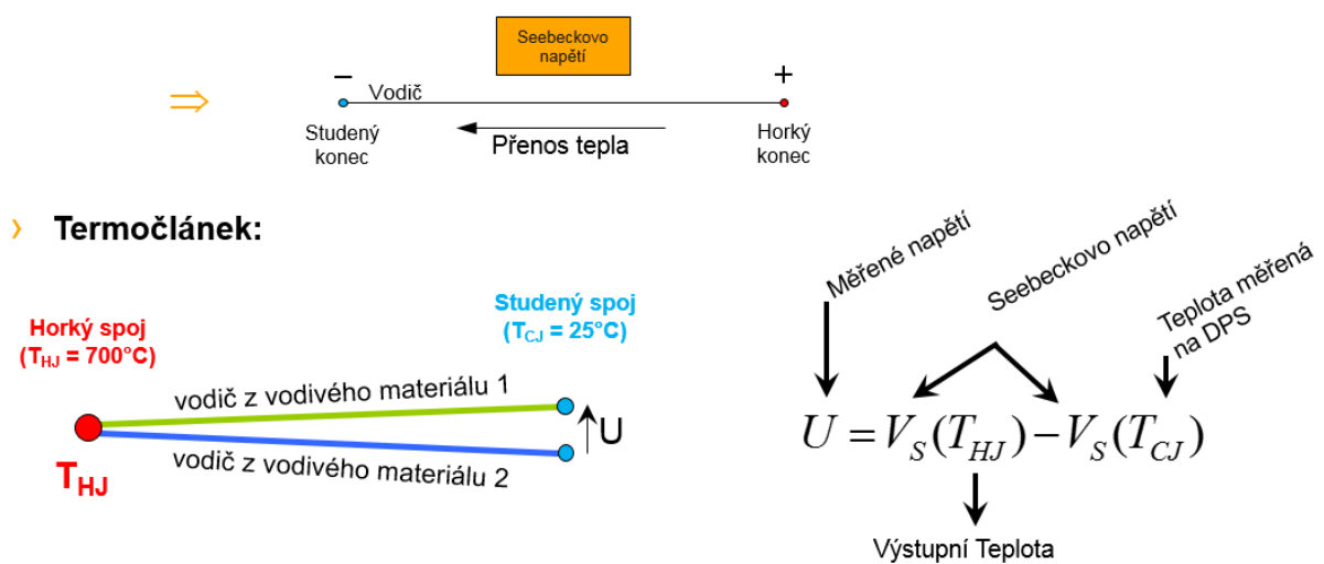
Obr. 6.3 Princip fungování termočlánku
