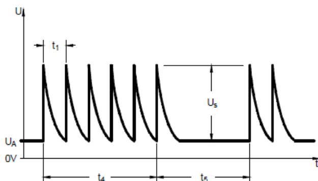
Obr. 11.4 Transientní pulzy
