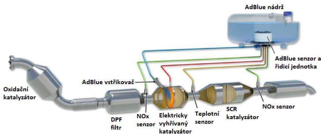
Obr. 7.8 Blokové schéma systému pro redukci oxidu dusíku
