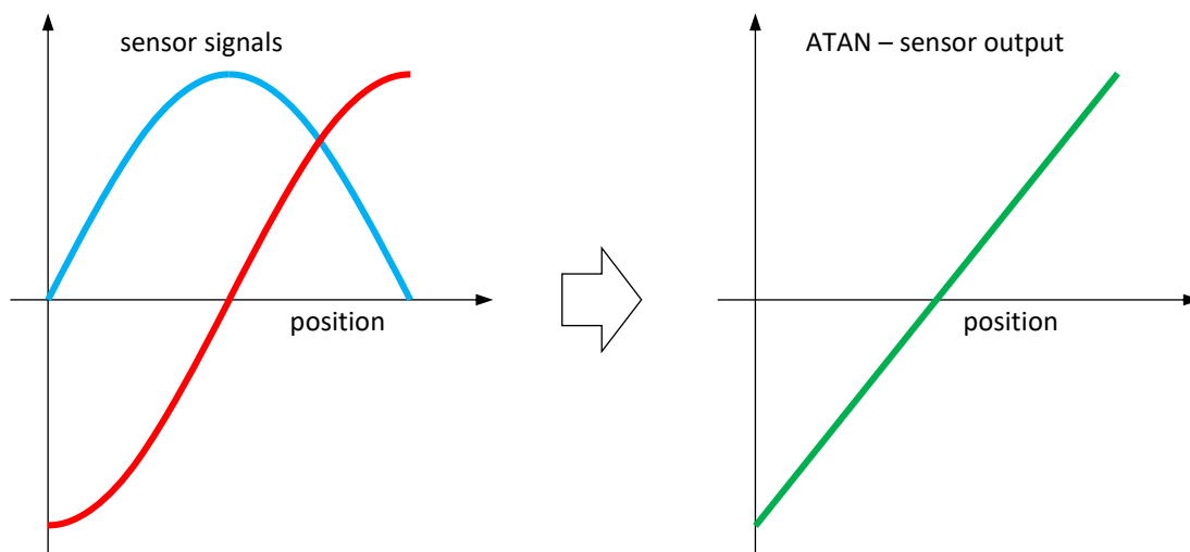
Obr. 8.6 Získání polohy z napětí jednotlivých Hallovyh snímačů
