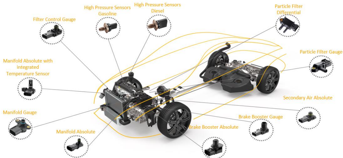
Obr. 9.4 Přehled a rozmístění tlakových senzorů v osobním automobilu
