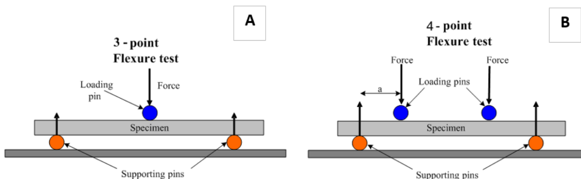
Obr. 5.2 Provedení zkoušky v ohybu (zobrazení tříbodové – A, čtyřbodové – B) [5.5]
