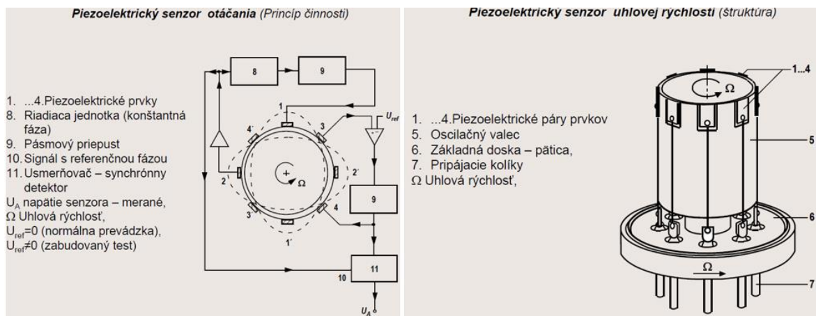
Obr. 9.10 Piezelektrické senzory otáčania a uhlovej rýchlosti [9.1]
