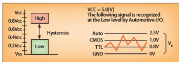
Obr. 12.2 Šum digitálního signálu [12.1]
