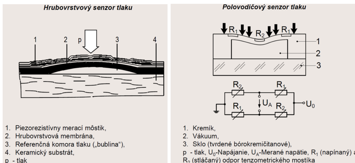
Obr. 9.2 Tlustovrstvý a polovodičový senzor tlaku [9.1]
