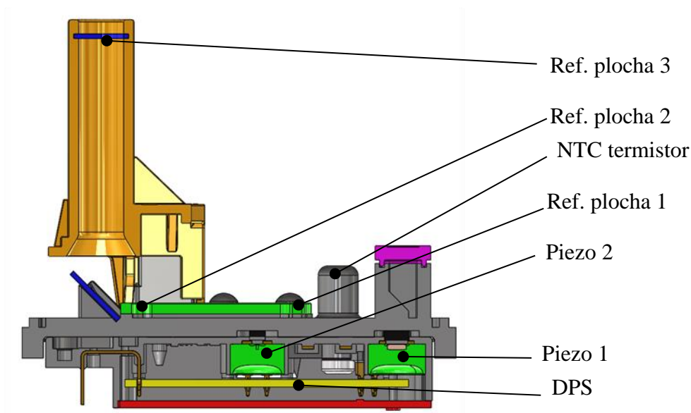
Obr. 7.10 Řez senzorem
