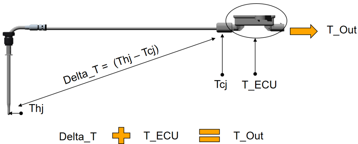
Obr. 6.5 Měřicí princip termočláňku vyráběného společností Vitesco Technologies
