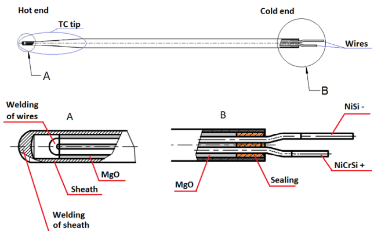
Obr. 6.4 Schematické znázornění termočláňku vyráběného společností Vitesco Technologies
