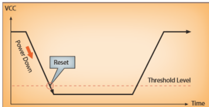
Obr. 12.1 Detekce nízkého napětí (Low voltage detection) [12.1]
