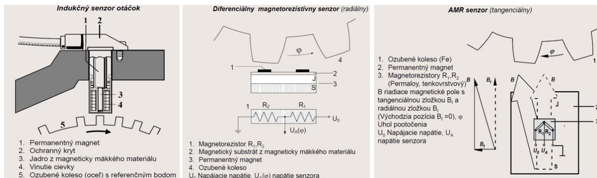
Obr. 9.9 Ukázka indukčného, gradientného a tangenciálneho snímače [9.1]
