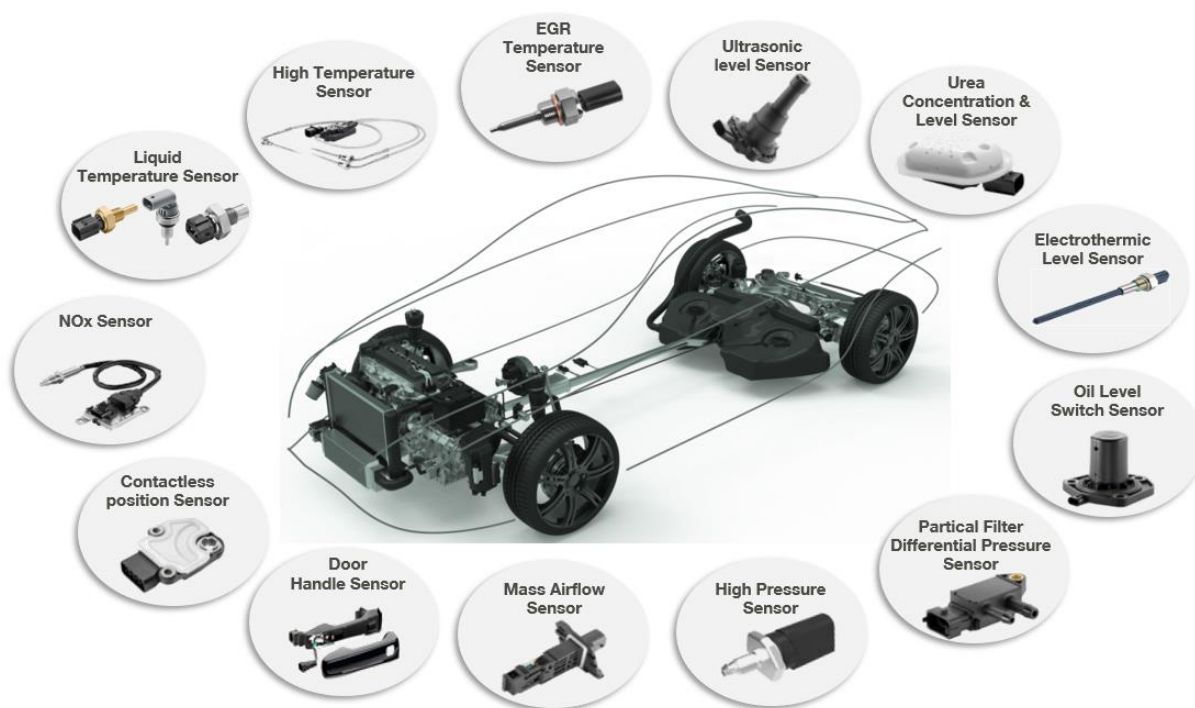
Obr. 2.2 Portfolio senzorů vyvíjených v lokaci Ostrava
