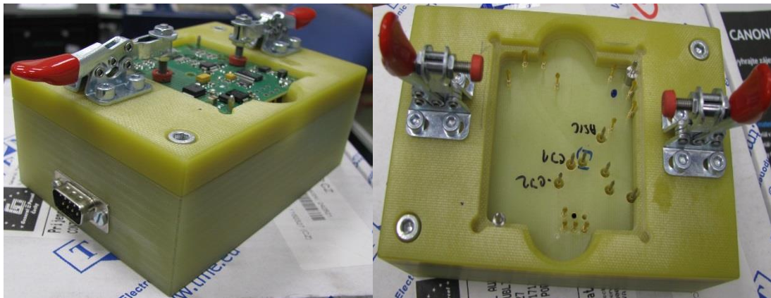
Obr. 11.10 Adaptér s kontaktními jehlami
