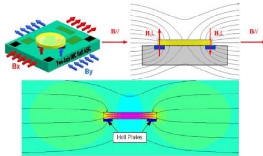
Obr. 8.5 Princip snímání pozice s využitím dvou Hallovyh snímačů magnetického pole
