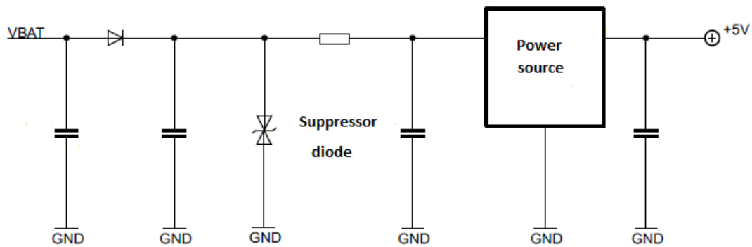
Obr. 11.6 Ochrana blokováním
