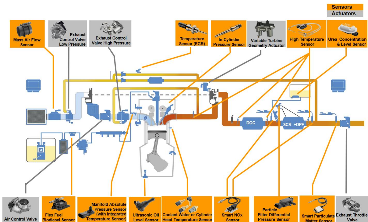
Obr. 2.6 Přehled senzorů a aktuátorů nacházejících se v oblasti motoru automobilu
