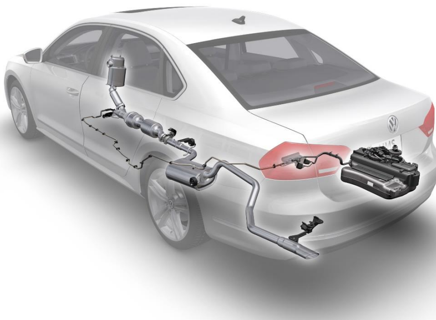
Obr. 7.9 Umístění systému redukce oxidu dusíku ve vozidle [7.6]
