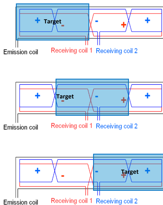
Obr. 8.9 Princip indukčního snímače pozice
