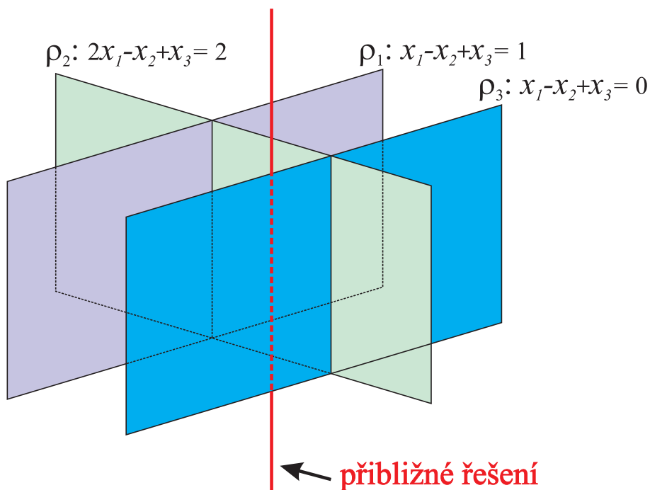
Obrázek 2.1: Jednotlivé rovnice soustavy jsou rovnicemi rovin v E_3 . Najít řešení soustavy znamená najít jejich společný průsečík. První rovnice a třetí rovnice jsou rovnicemi rovnoběžných rovin, které se neprotínají. Proto soustava nemá řešení. Přibližným řešením získaným pomocí metody nejmenších čtverců je množina bodů (tvoří přímku), které jsou „co nejbliž“ všem třem rovinám.
